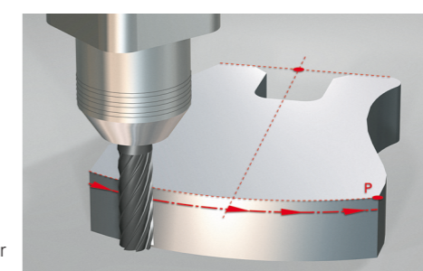
CHF Fase: Angabe des Eckpunktes und der Faselänge
