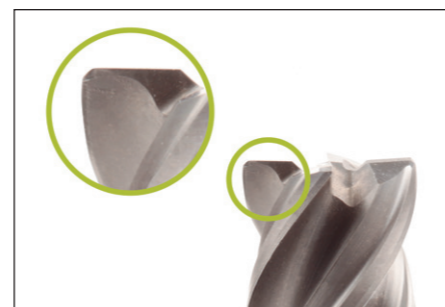
Bearbeitung mit OCM: Werkzeug nach 6 Teilen
