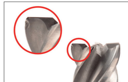
Bearbeitung ohne OCM: Werkzeug nach 2 Teilen
